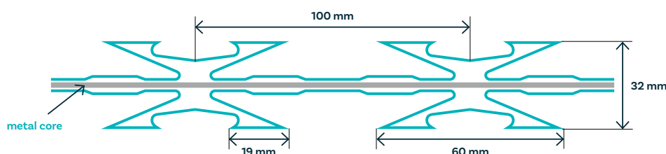
CBT 60 dimensions
