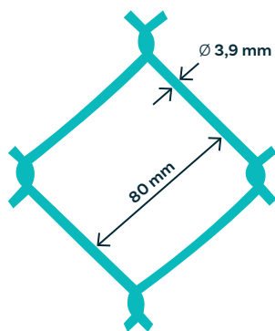
Schéma de la maille
