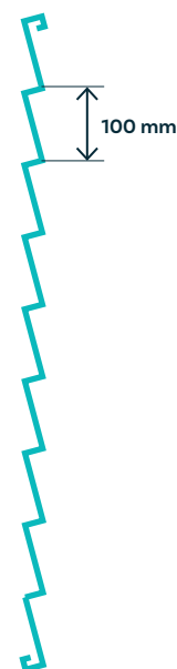
Clôture standard Clins 100 mm
