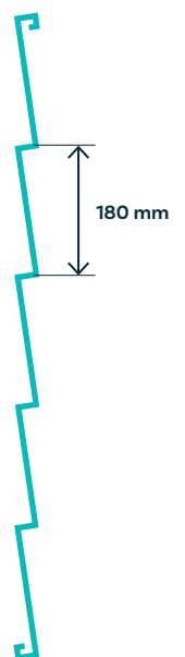
Clôture XL Clins 180 mm
