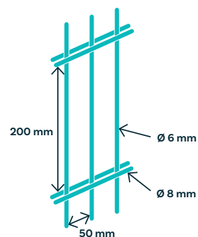
Panneau Ø 8/6/8
